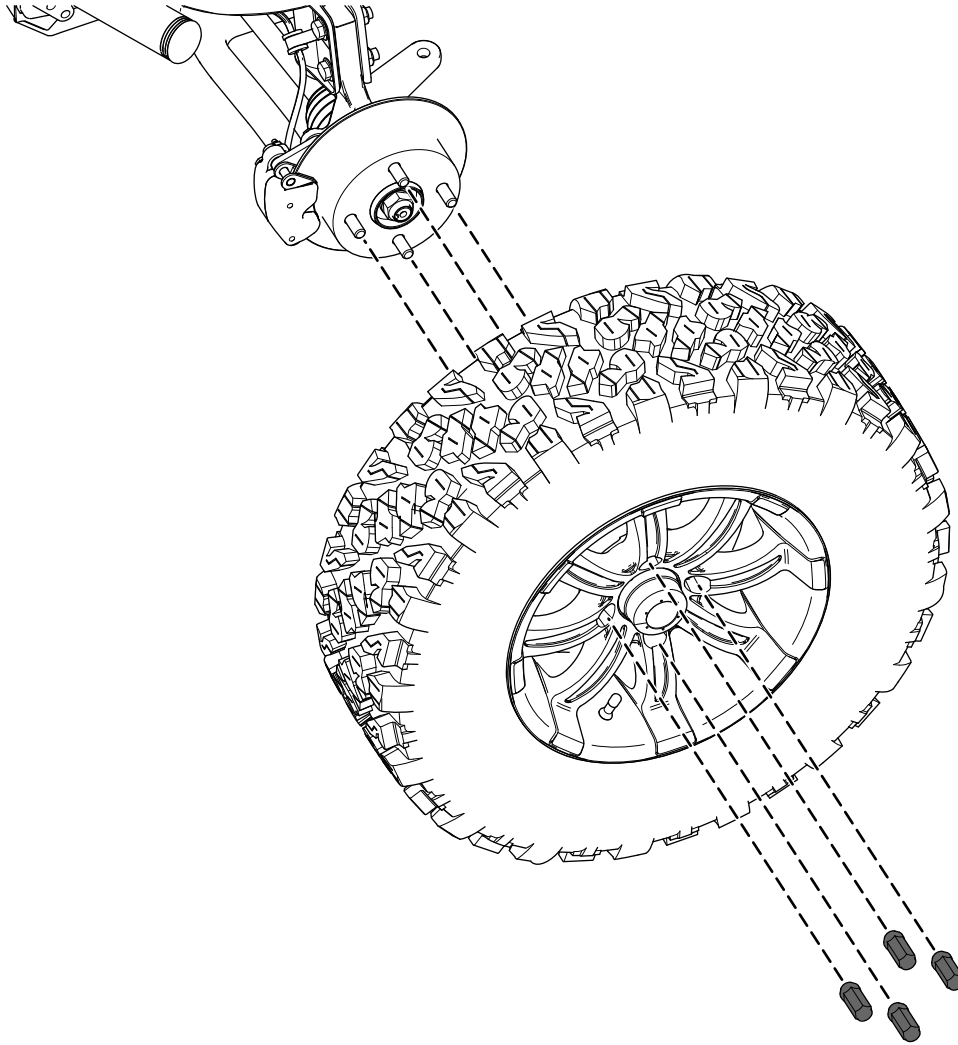
Kuvassa vasen etupyöräkokooppa
