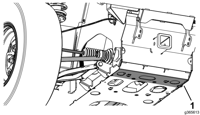
1. Donkraftpunkt foran
