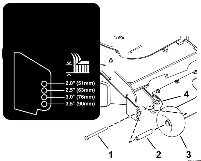
Ábra 29 Hátsó kidobású gépek
