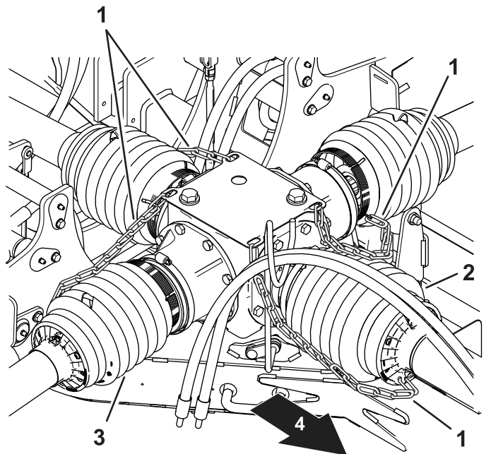
Figur 18 Mittväxellåda
