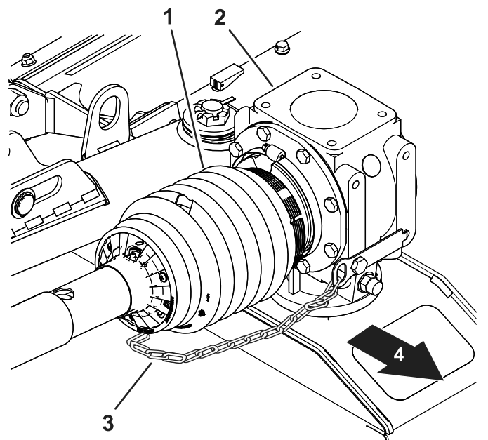
Figur 19 Vänstra klippdäckets drivaxelskydd
