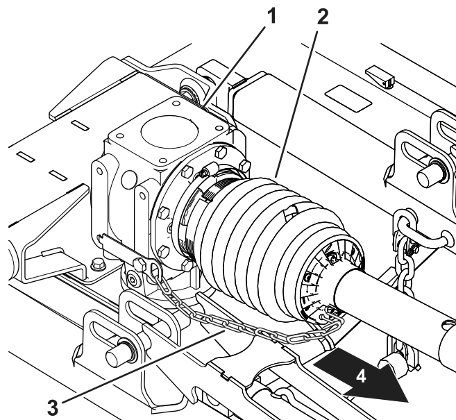
Figur 20 Mittklippdäckets drivaxelskydd
