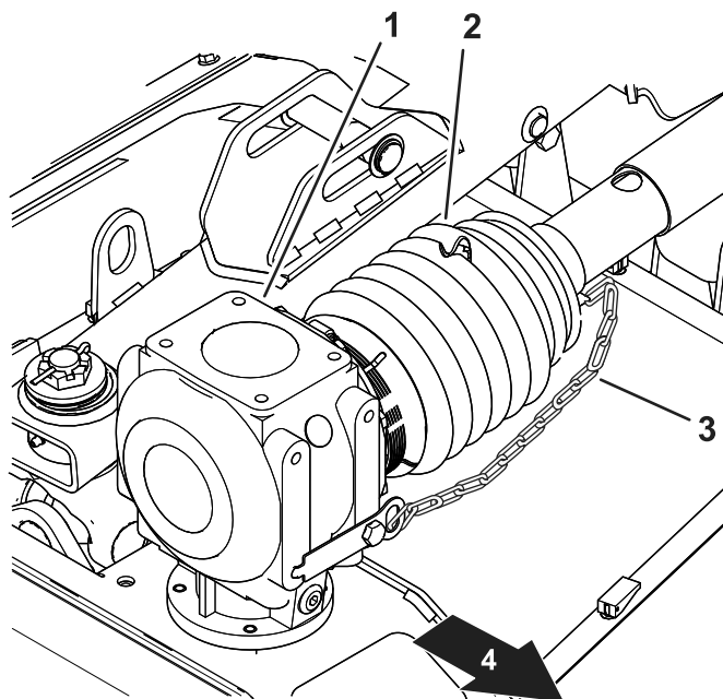
Figur 21 Högerklippdäckets drivaxelskydd
