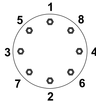
Figur 21 Framhjul
