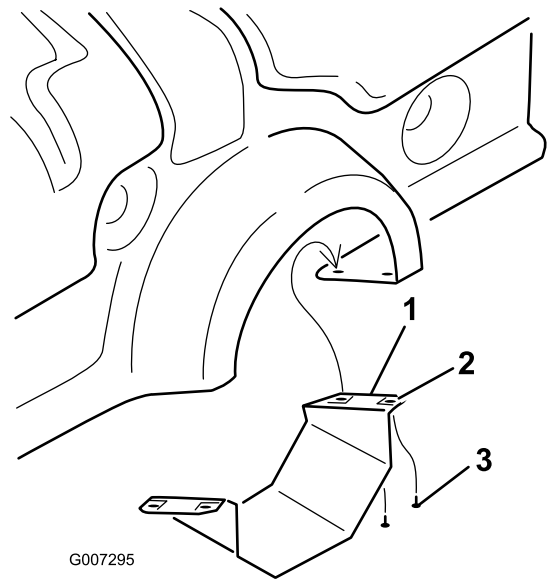
Figura 10 ProCore 864
