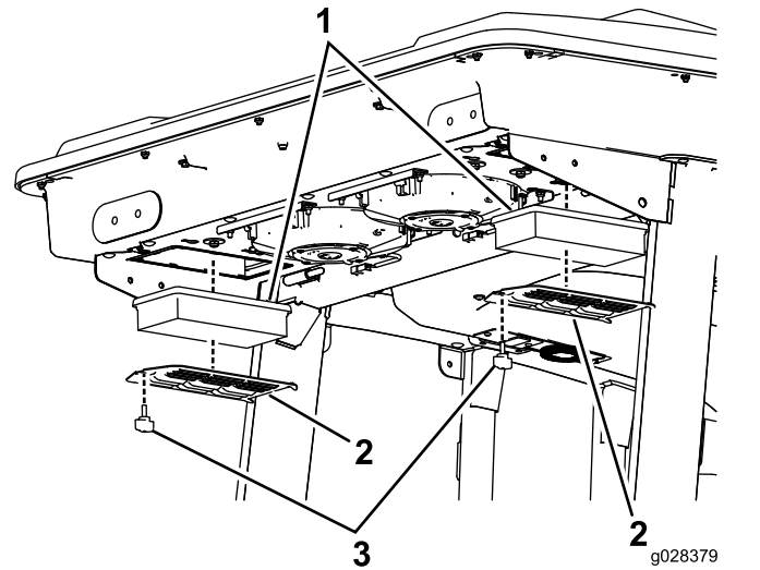
Figure 146 Filtre à air arrière de la cabine
