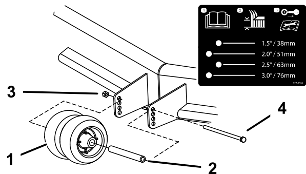
Figur 12 Frontruller vist
