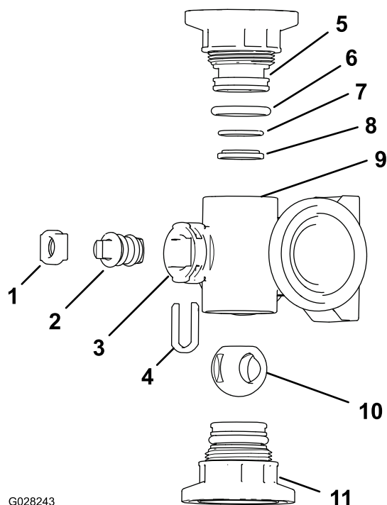
图 110 搅拌阀歧管
