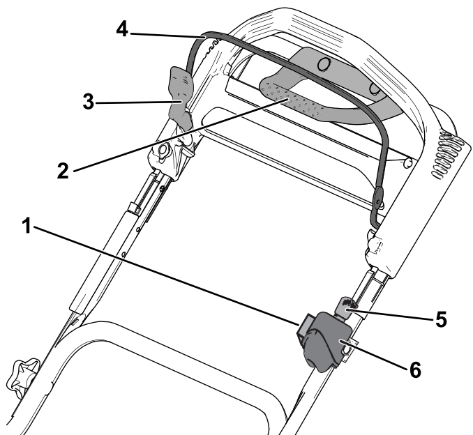
Figura 8 Manillar superior
