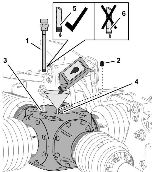
Bild 61 Zentralgetriebe
