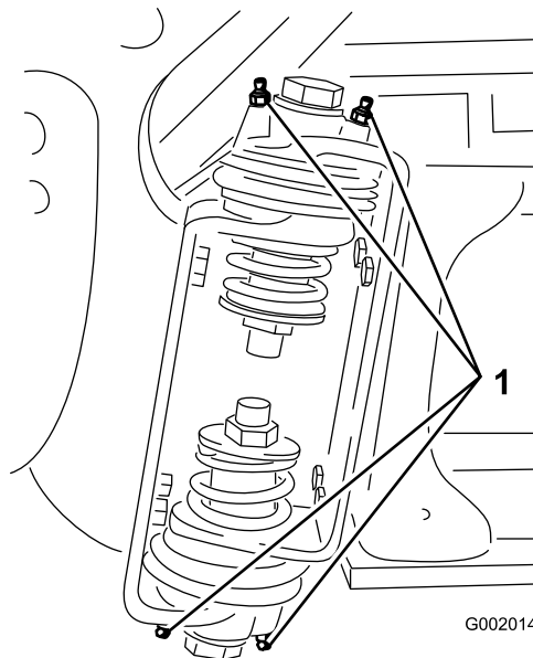
图35 右喷洒臂
