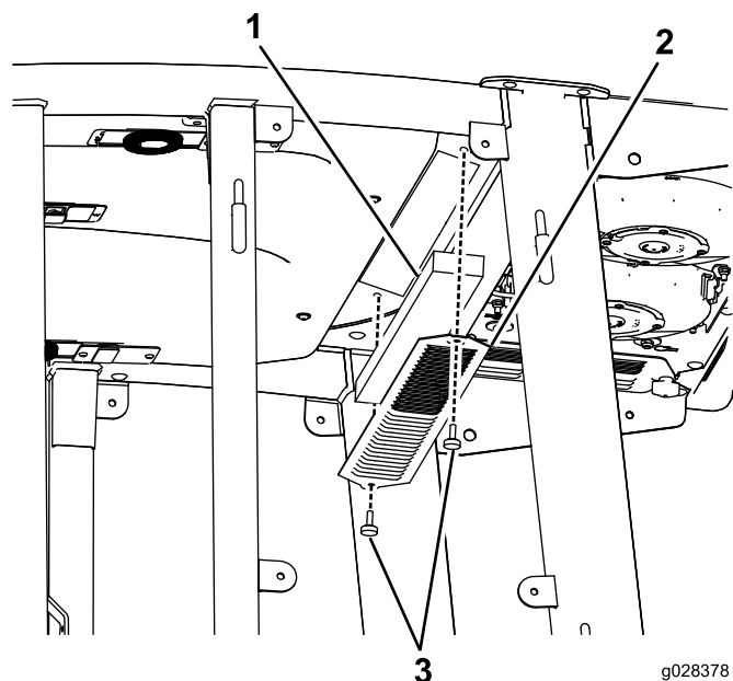
Figur 115 Luftfilter i førerhus
