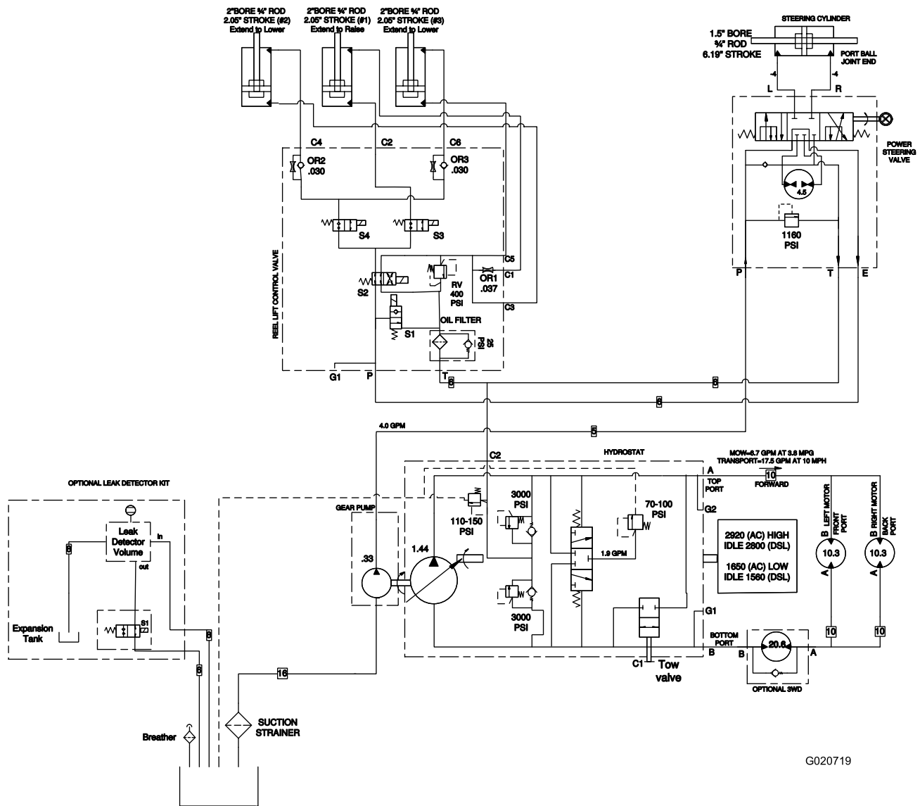
Hydraulischaltplan (Rev. A)
