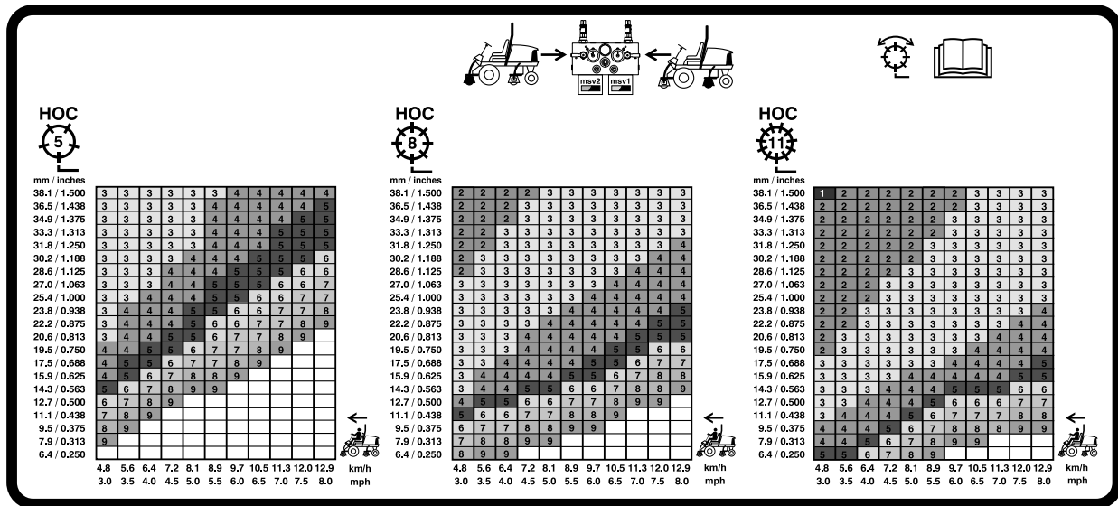
Figura 60 Tabella della velocità dei cilindri 127 mm
