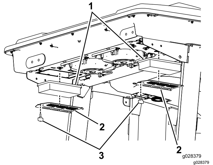
Figuur 114 Luchtfilter achter de cabine
