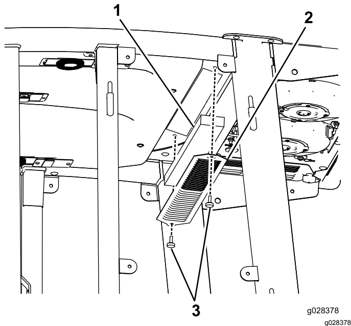
Figuur 113 Luchtfilter in de cabine
