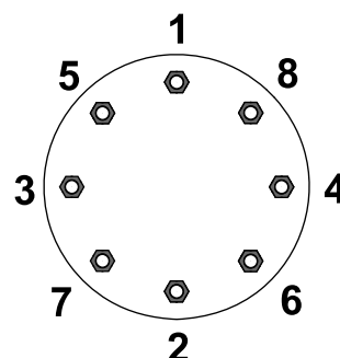
Figur 14 Framhjul
