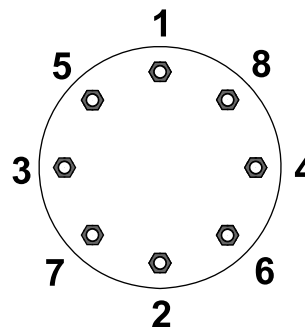
Figure 12 Roues avant
